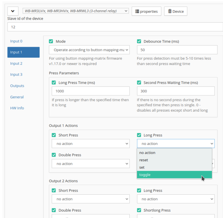
Рис. 12. Привязка действий к типам нажатий
