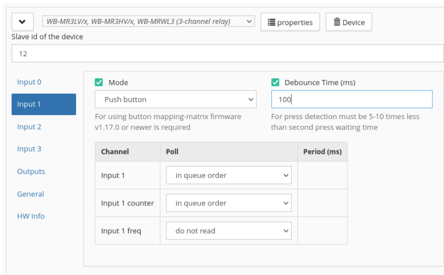
Рис. 13. Пример установки времени антидребезга
