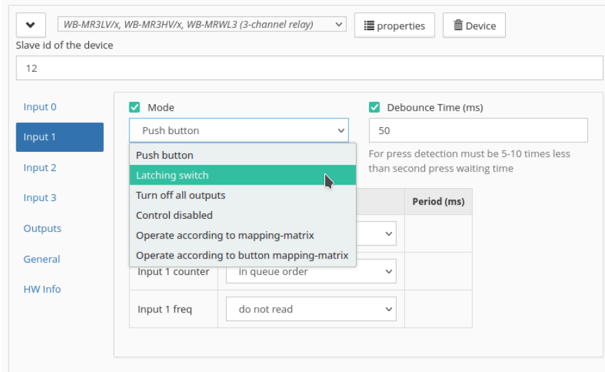
Рис. 11. Выбор режима для 1 входа реле
