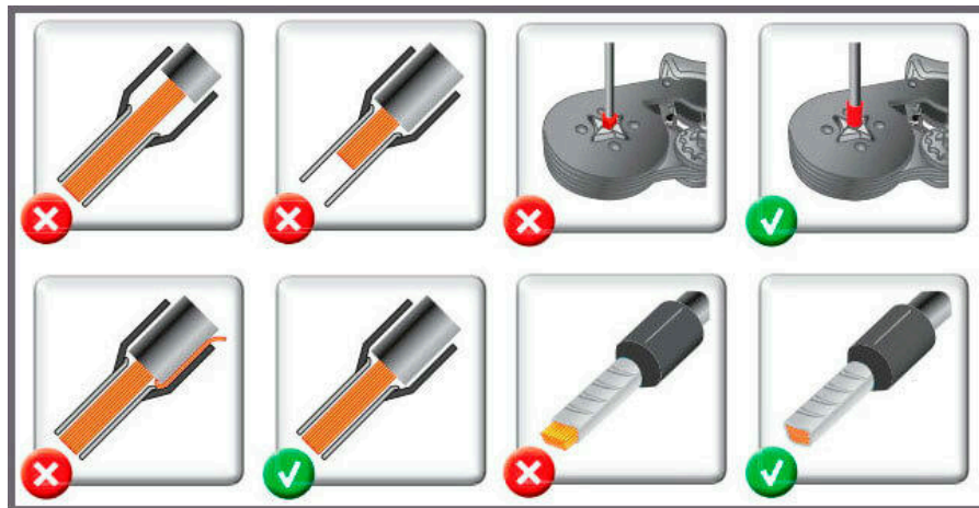
Рис. 5. Как обжимать наконечники НШВИ
