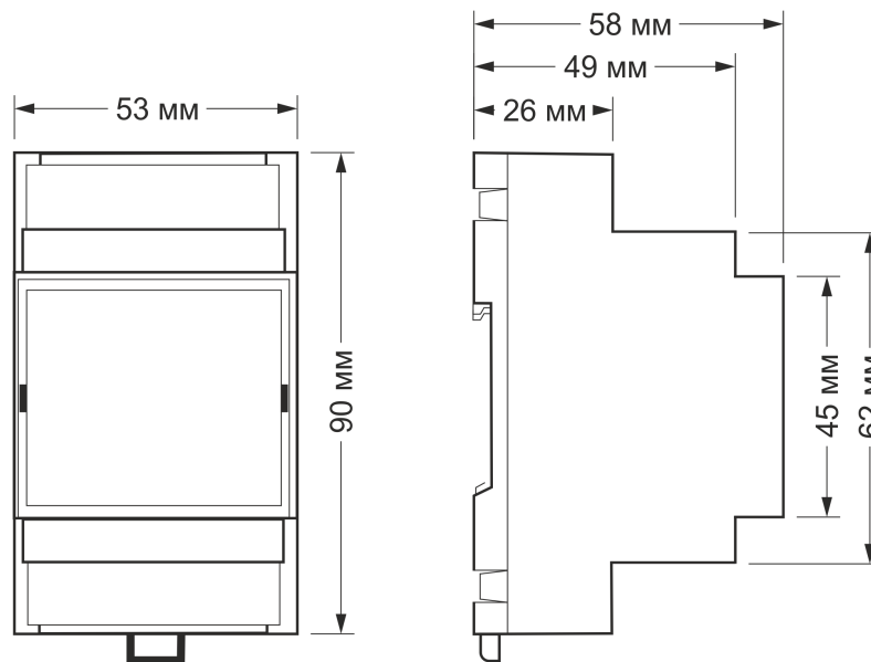
Рис. 27. Габаритные размеры WB-MRWL3 составляют 53,3 x 90,2 x 57,5 мм (Д x Ш x В)
