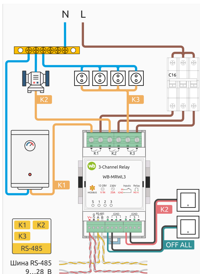
Рис. 6. Пример монтажа WB-MRWL3
