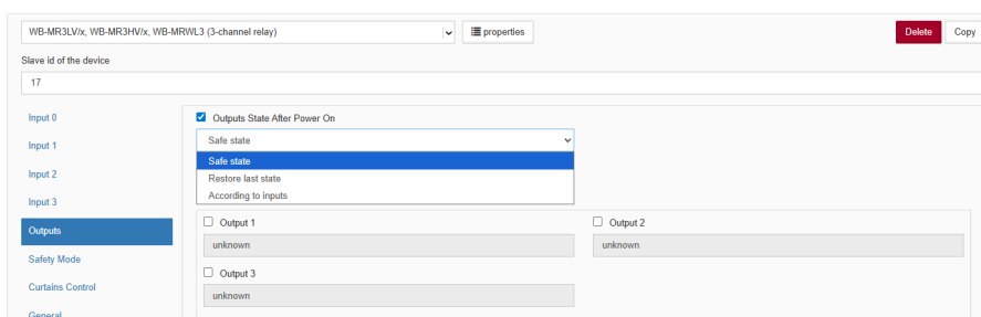
Рис. 14. Настройка состояния реле при подаче питания
