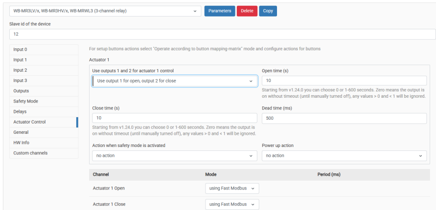
Рис. 17. Примеры настройки модуля для работы с приводом. Настройка режима управления приводом для выходов K1 и K2
