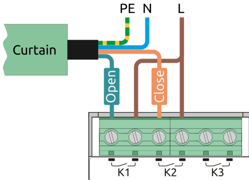
Рис. 7. Пример подключения привода штор к модулю WB-MRWL3
